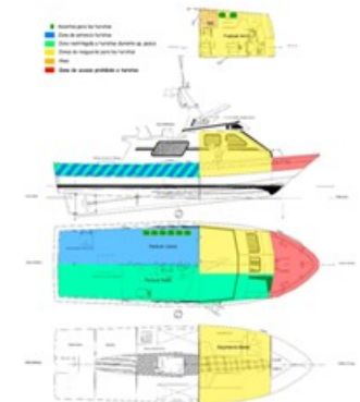
Figura 10- Plano de la embarcación con definición de zonas
